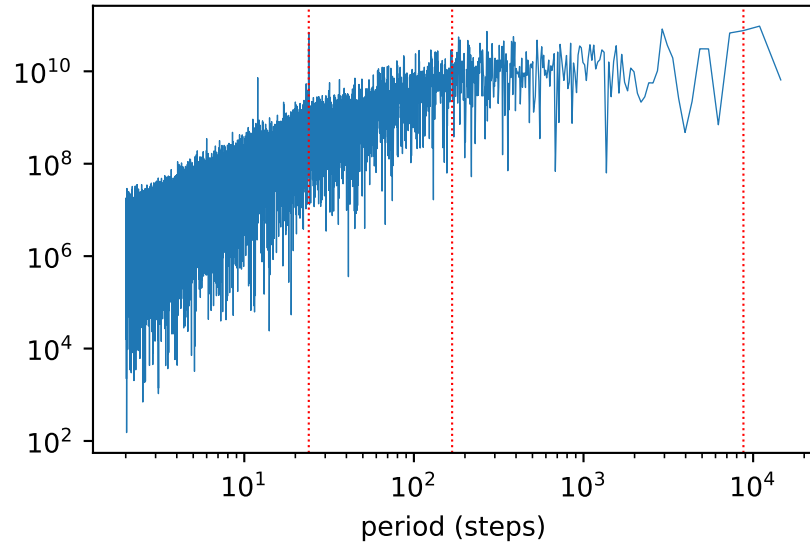
Periodogram
