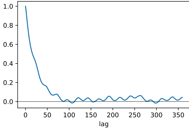
ACF
